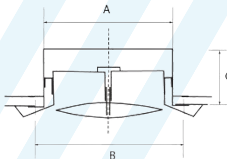
DIMENSIONI SEZIONE
