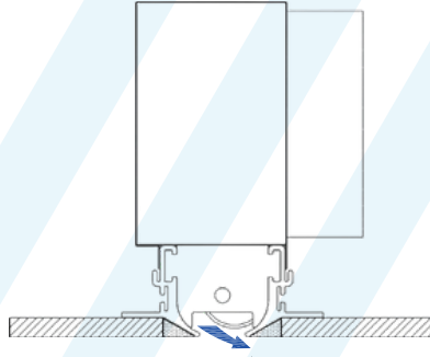
CONFIGURAZIONE B LANCIO VERSO SINISTRA
